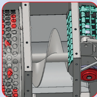
SISTEMA DI PULIZIA SUPPLEMENTARE CON SEPARATORI E DERASPATORI INTEGRATI NELLE VASCHE
